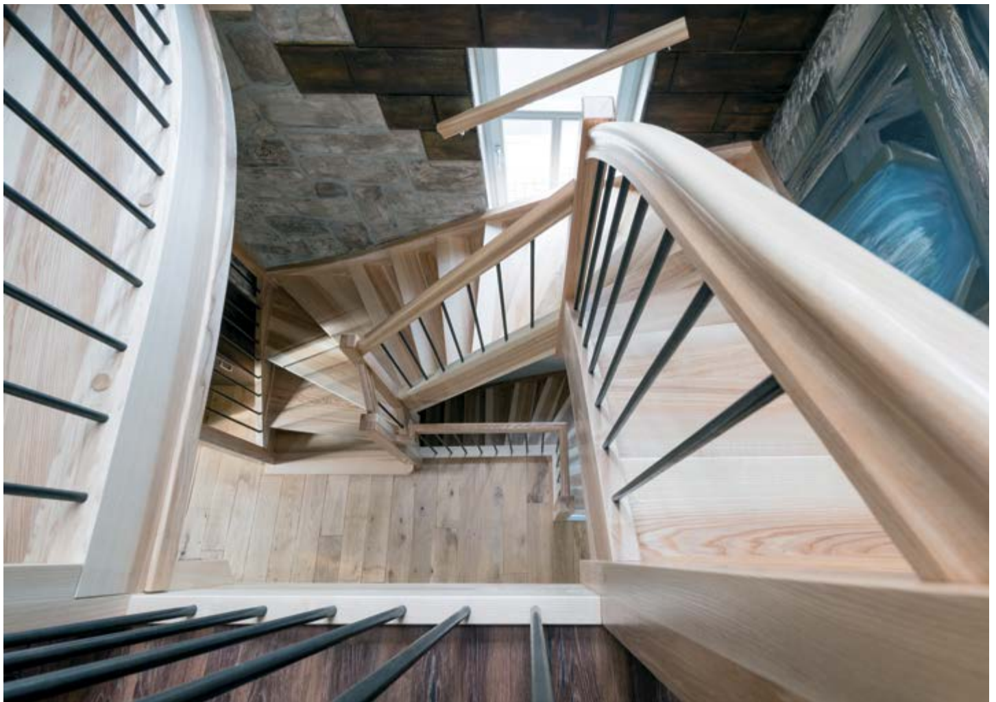
Wangentreppe COMFORTLINE aus Esche MB gefertigt, Stäbe aus Schwarzstahl, Handlauf als Omegahandlauf in geschwungener Ausführung, Oberfläche lackiert.
