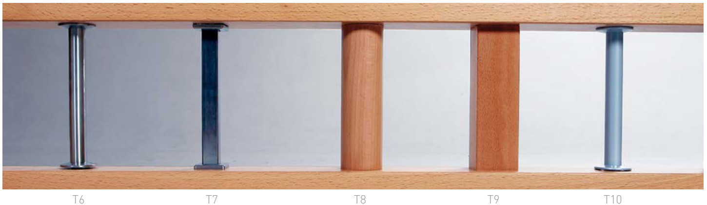
Tragbolzen für BasicLine- sowie StandardLine-Treppen
